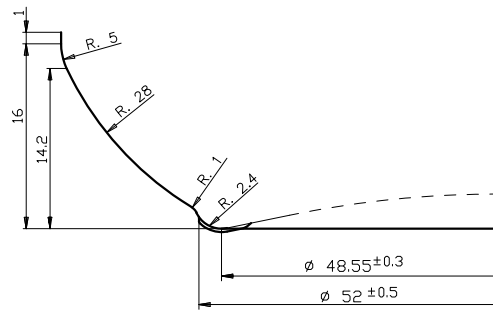
PARTICOLARE GRADINO DI IMPILAGGIO Scala 3:1
